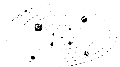
le système solaire
